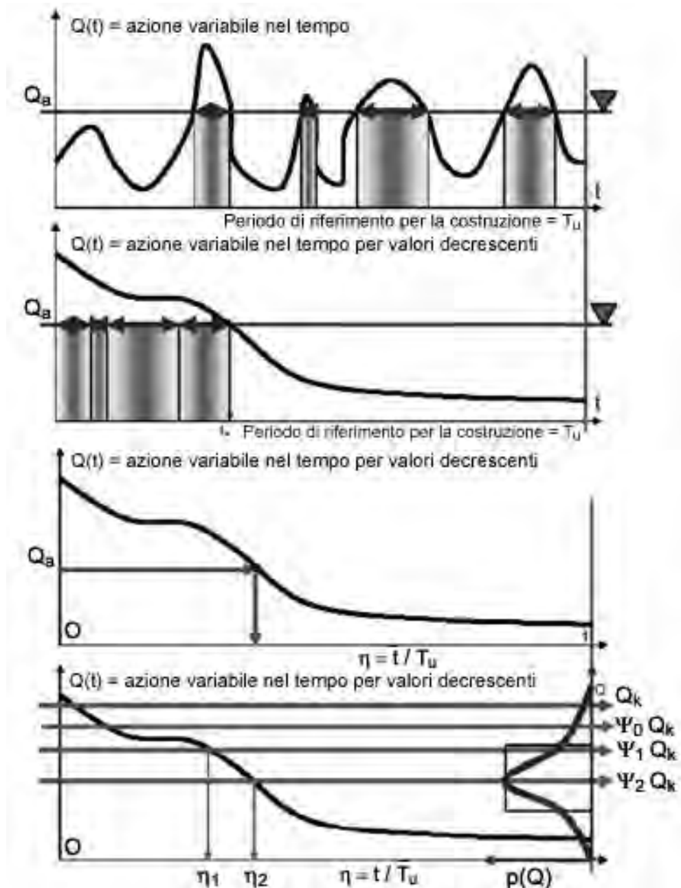
Figura 2.6.1 - Modalità di descrizione di una azione variabile nel tempo
