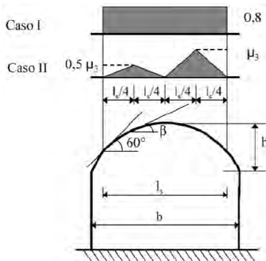
Figura 3.5.7 - Disposizioni di carico per coperture cilindriche
