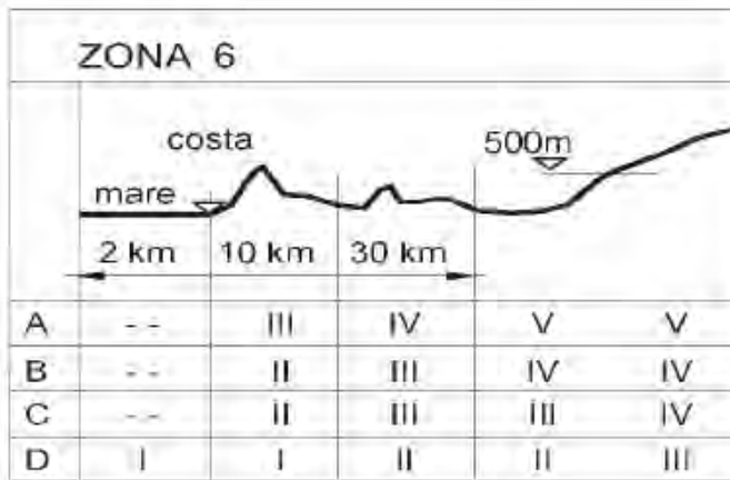
Figura 3.3.3 - Definizione delle categorie di esposizione I, II, III, IV e V, in funzione delle regioni individuate nella macrozonazione
