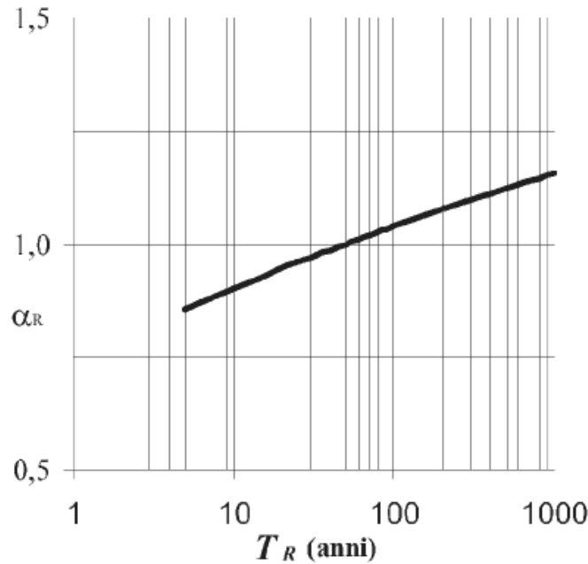
Figura 3.3.2 - Valori del coefficiente \alpha_R per la definizione della velocità di riferimento del vento in funzione dei periodo di ritorno T_r
