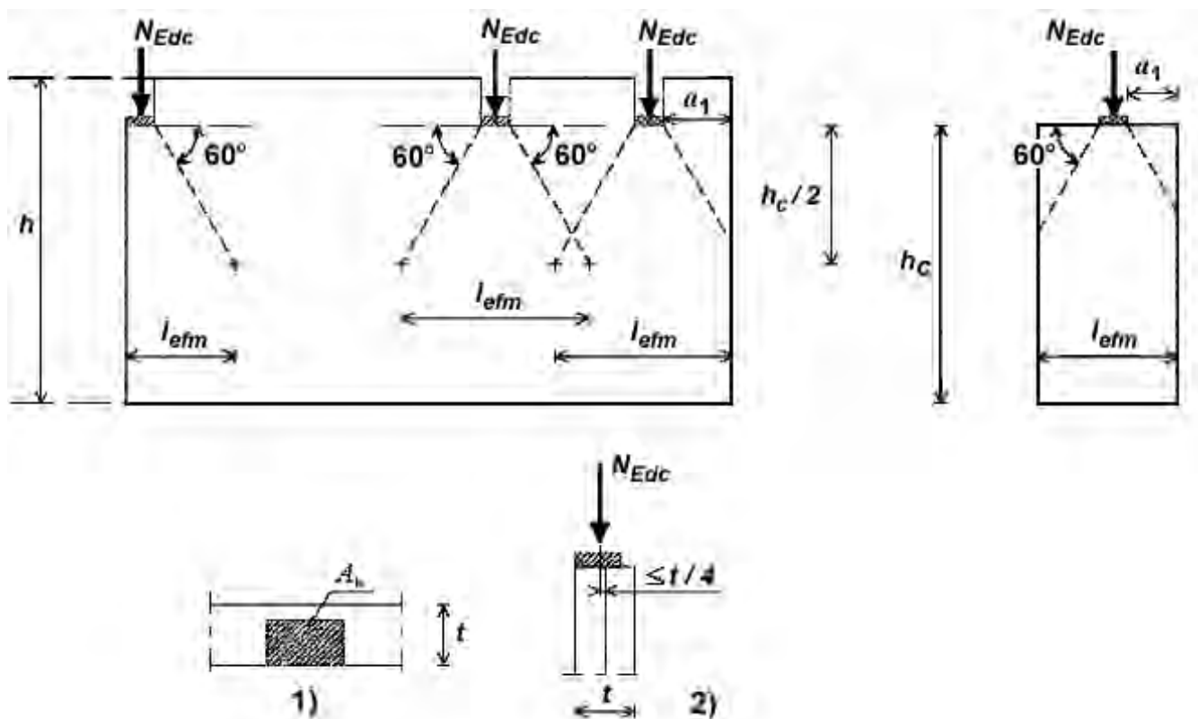
Figura 5.4.1. - Pareti soggette a carichi concentrati. 1) pianta, 2) sezione
