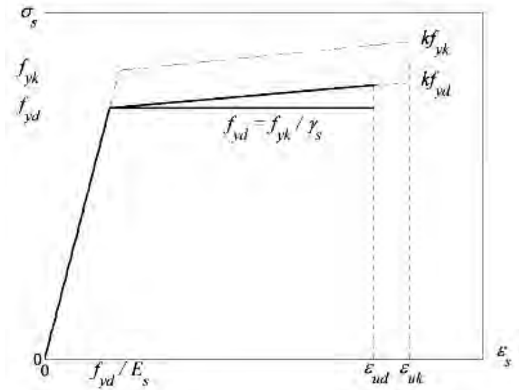
Figura 5.1.2. - Diagrammi di calcolo tensione/deformazione per l'acciaio (linee continue) e diagramma caratteristico (linea tratteggiata)
