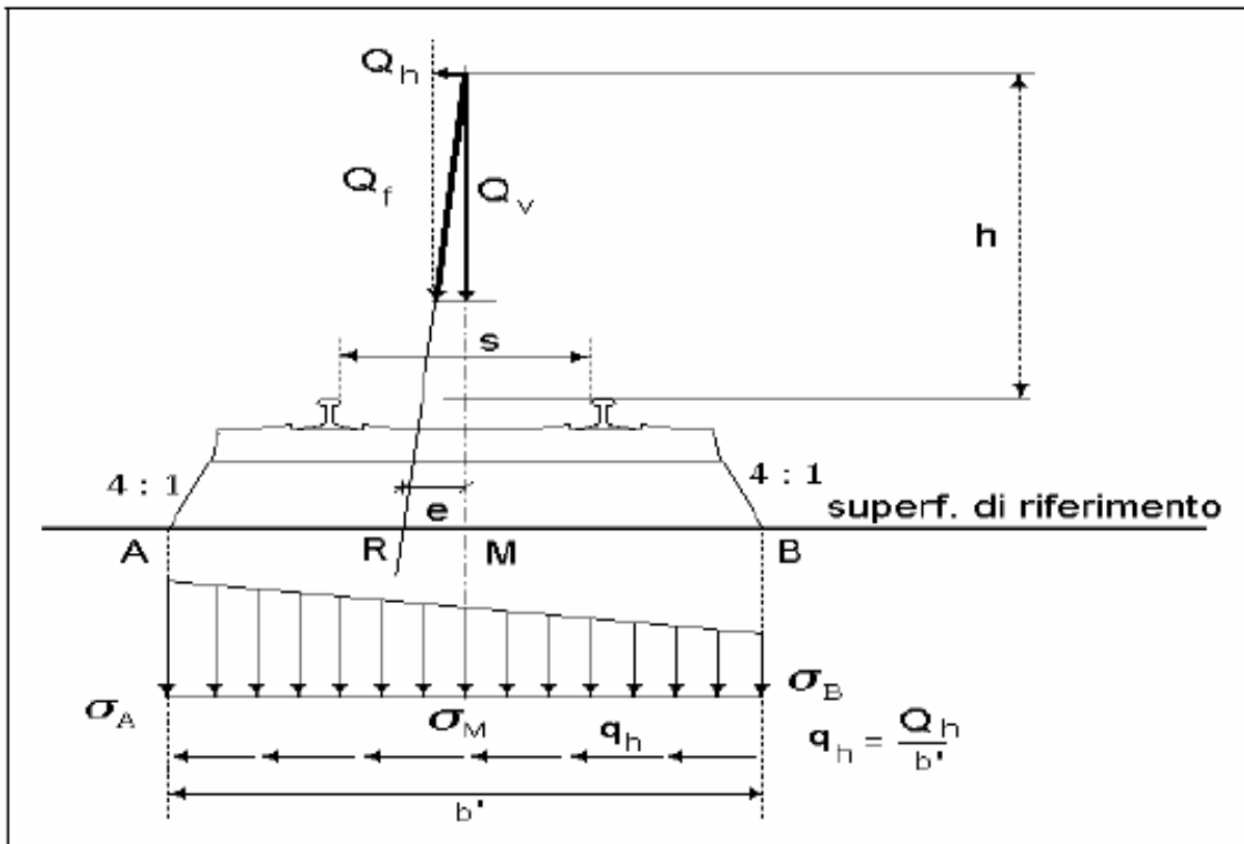
Figura 6.3.5 - Distribuzione trasversale in rettifilo delle azioni per mezzo delle traverse e del ballast
