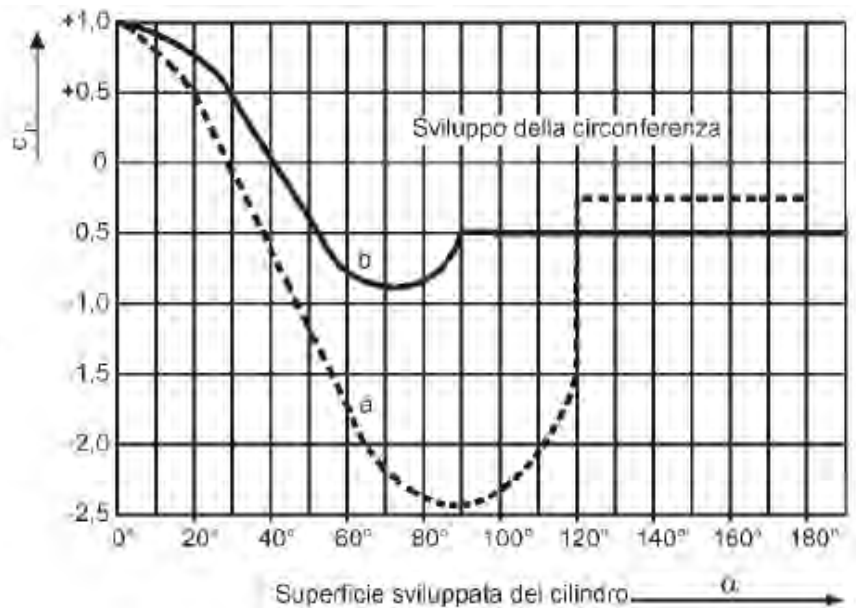
Figura 3.3.12 - Coefficienti di pressione esterna delle superfici cilindriche e sferiche: curva (a) per superfici lisce (metalli, intonaco liscio); curva (b) per superfici ruvide (muratura con giunti di malta, intonaco rustico)
