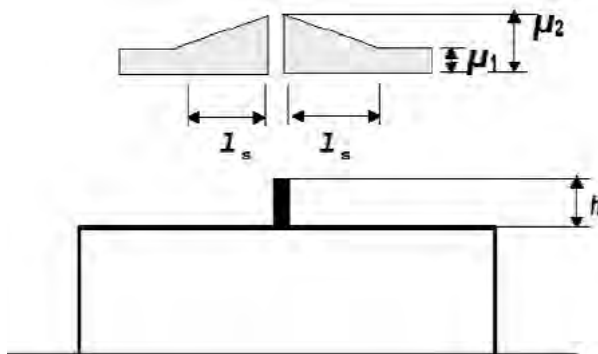
Figura 3.5.10 - Coefficienti di forma in prossimità di parapetti e pareti verticali
