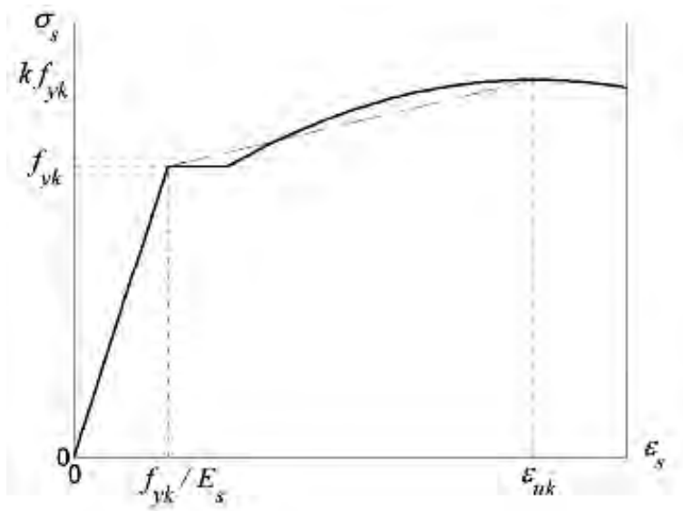
Figura 5.1.3. - Diagramma tensione/deformazione per acciaio a snervamento definito (linea continua) e relativo diagramma caratteristico (linea tratteggiata)
