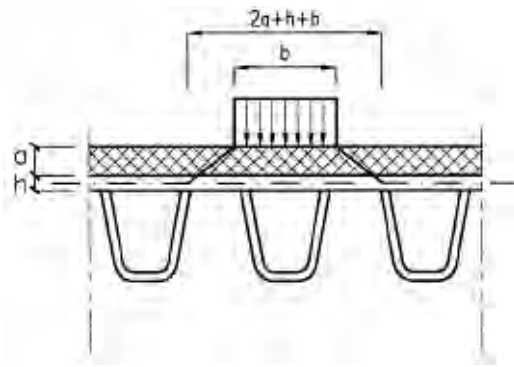
Figura 6.2.3b - Diffusione dei carichi concentrati attraverso la pavimentazione e gli impalcati a piastra
